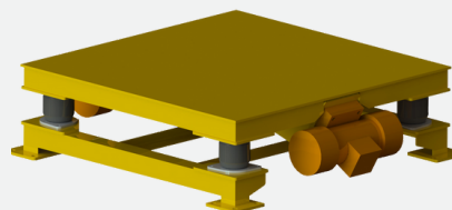
Vibrační stůl
